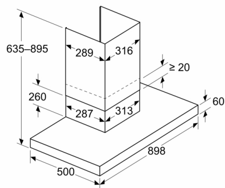
Afmeting in mm Apparaat in luchtafvoermodus
